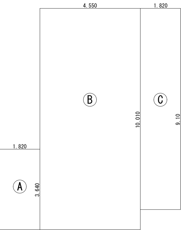
建築面積求積図 S=1/100
